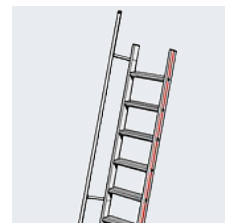
Corrimão Em tubo de alumínio Ø 30 mm, com ranhura em T, para mudar a posição. Afastamento de 150 mm ao montante
